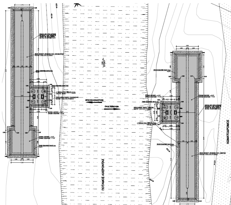
ΟΡΙΖΟΝΤΙΟΓΡΑΦΙΚΗ ΔΙΑΤΑΞΗ ΘΕΜΕΛΙΩΣΗΣ ΦΟΡΕΑ ΠΕΖΟΓΕΦΥΡΑΣ & ΤΕΧΝΙΚΩΝ ΠΡΟΣΒΑΣΗΣ
