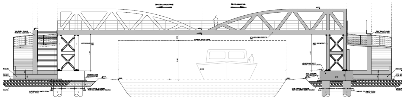
ΟΨΗ ΦΟΡΕΑ ΠΕΖΟΓΕΦΥΡΑΣ
