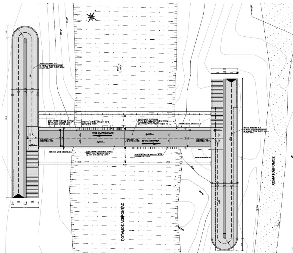
ΔΙΑΤΟΜΗ ΦΟΡΕΑ ΚΑΤΑΣΤΡΩΜΑΤΟΣ ΣΕ ΘΕΣΗ ΣΤΗΡΙΞΗΣ
