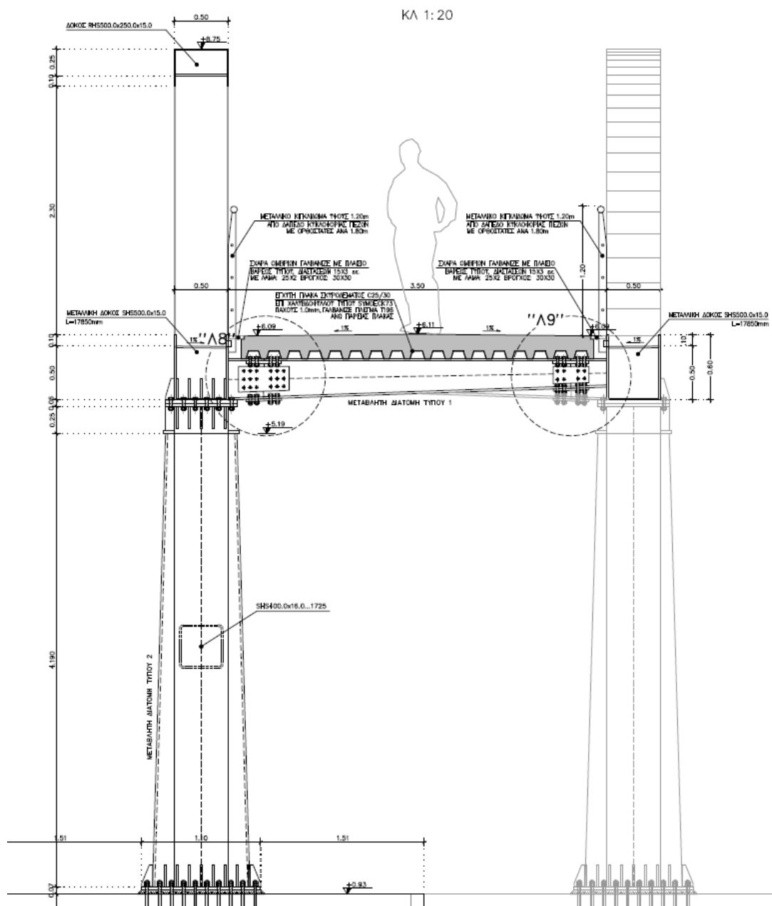
ΚΑΤΑ ΠΛΑΤΟΣ ΤΟΜΗ ΚΑΤΑΣΤΡΩΜΑΤΟΣ ΠΕΖΟΓΕΦΥΡΑΣ ΣΕ ΘΕΣΗ ΕΔΡΑΣΗΣ
